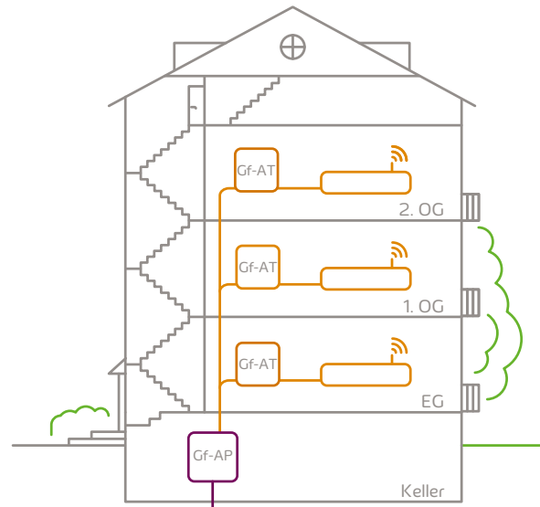
Gf-AP: Glasfaser-Abschlusspunkt | Gf-TA: Glasfaser-Teilnehmeranschlussdose
