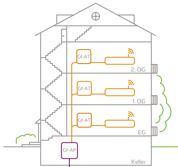
Gf-AP: Glasfaser-Abschlusspunkt | Gf-TA: Glasfaser-Teilnehmeranschlussdose
